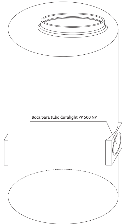
PERSPECTIVA
