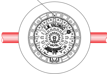
Tampa em ferro fundido dúctil D400 Ø800mm
