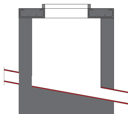
Corte
