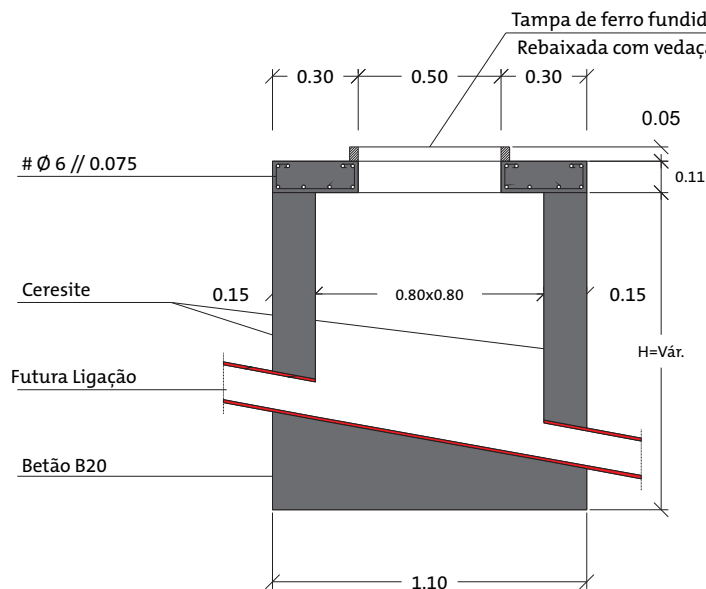
Corte
