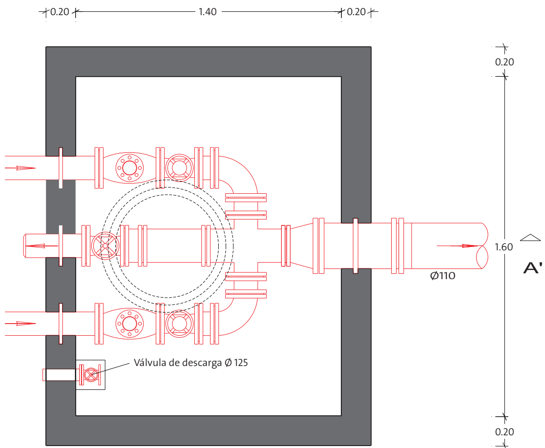
Planta
